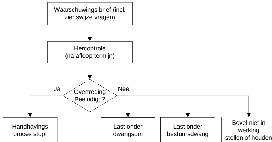
Schema reactie 2
